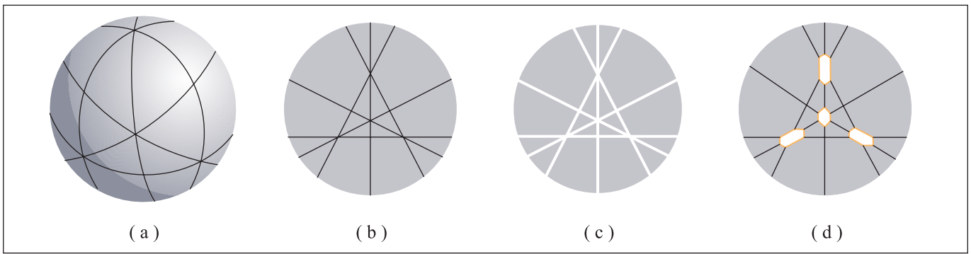
Figure 9. (a) SV^2 , (b) PV^2 , (c) PV^2_{gf} , and (d) PV^2_{\#} .
